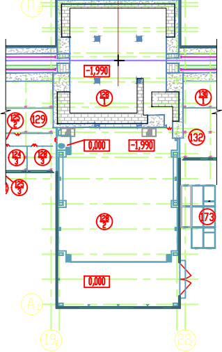
Компоновка здания N17. M1:500. План на отм. 0,000 II пусковой комплекс
