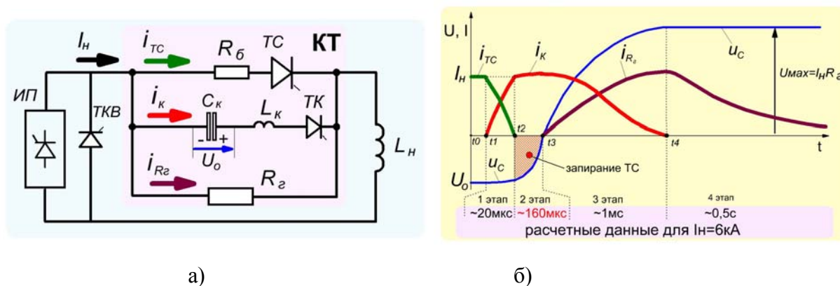
Рис. 4 Схема ключа эвакуации а) и коммутационные процессы при эвакуации энергии б). ИП – источник тока, ТКВ – тиристорный замыкатель, ТС – тиристор силовой, Rб – балластный резистор, ТК – тиристор коммутационный, Ск – конденсатор, Uо – напряжение предварительного заряда Ск , Lк – коммутационная катушка, Rг – резистор гашения поля, Lн – индуктивность нагрузки.
