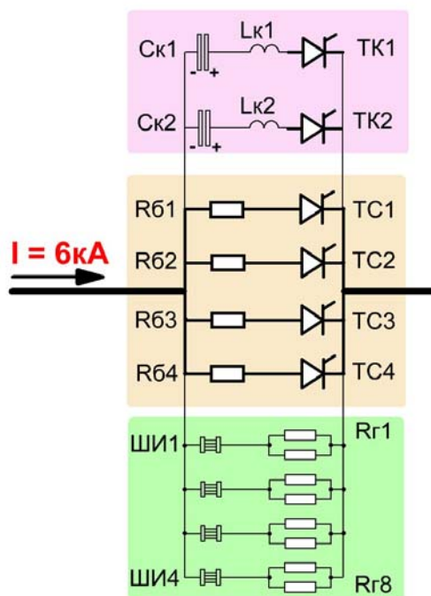
Рис. 5. Принципиальная схема ключа эвакуации энергии КТ. C_{к1}=C_{к2} – конденсаторная батарея 6мФ \times 1000В , L_{к1}=L_{к2} – коммутационная катушка 3мкГн , TC1..4 – тиристор силовой типа ТБ373-2000-20, TK1,2 – тиристор коммутационный типа ТБ373-2000-20, R_{б1}...4 – балластный резистор типа РКш173-000,5 номиналом 0,5мОм , R_{r1}...8 – резистор гашения поля типа Б8У2 номиналом 1,2Ом , ШИ1...4 – шунт измерительный типа 75ШИС-750.
