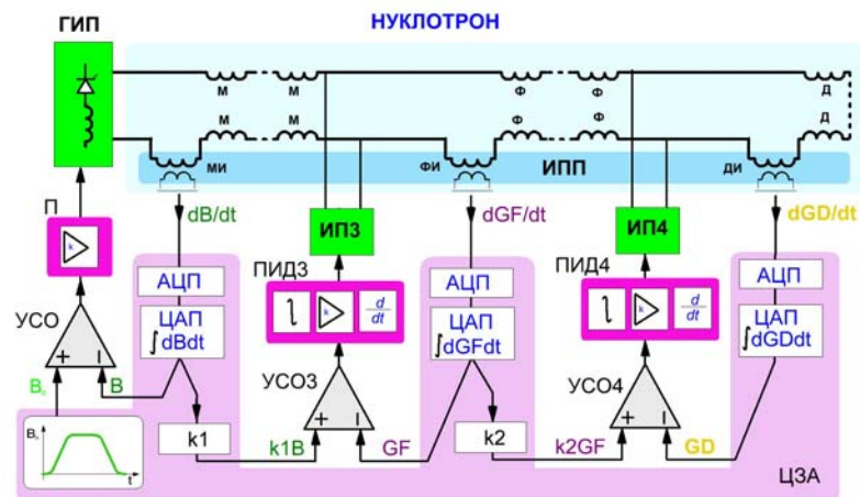
Рис. 3. Схема регулирования. ИПП – измерительный полупериод, ФИ - измерительная линза \Phi , GF – градиент поля \Phi линз, ДИ - измерительная линза D , GD – градиент поля D линз, МИ - измерительный магнит, V – поле дипольных магнитов, ЦЗА – цикло-задающая аппаратура, АЦП – аналого-цифровой преобразователь, ЦАП – цифро-аналоговый преобразователь, k – множительный усилитель, УСО – усилитель сигнала ошибки, ПИД – пропорционально-интегрально-дифференциальный регулятор, П - пропорциональный регулятор
