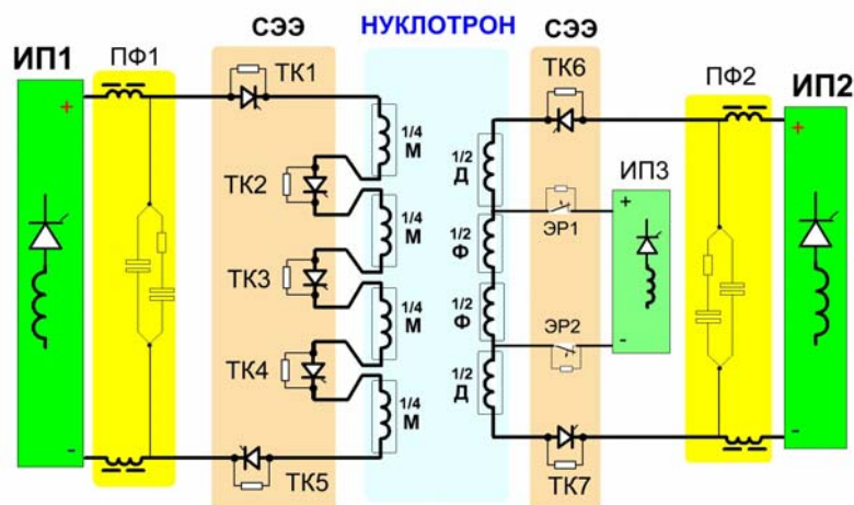
Рис.1. Принципиальная схема существующей системы питания. ИП – источник питания ПФ – пассивный фильтр, СУЭ – система эвакуации энергии, КТ – тиристорный ключ, ЭР – электронный размыкатель, М – дипольный магнит, Ф – фокусирующая линза, Д – декусирующая линза .
